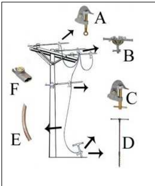
Figura 59 - Conjunto de aterramento temporário AT.
