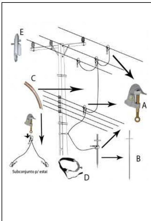
Figura 60 - Conjunto de aterramento temporário AT com sela.
